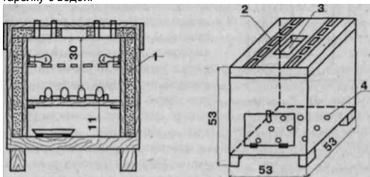
Рис. 25. Инкубатор простой конструкции: 1 — пространство между стенками; 2 — вентиляционные отверстия; 3 — окошко; 4 — отверстия пола
