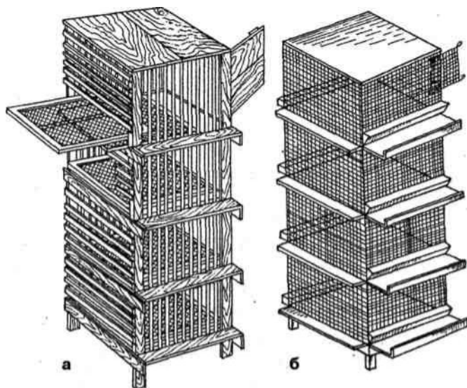
Рис. 15. Клетка для содержания перепелов: а — деревянная; б — металлическая
